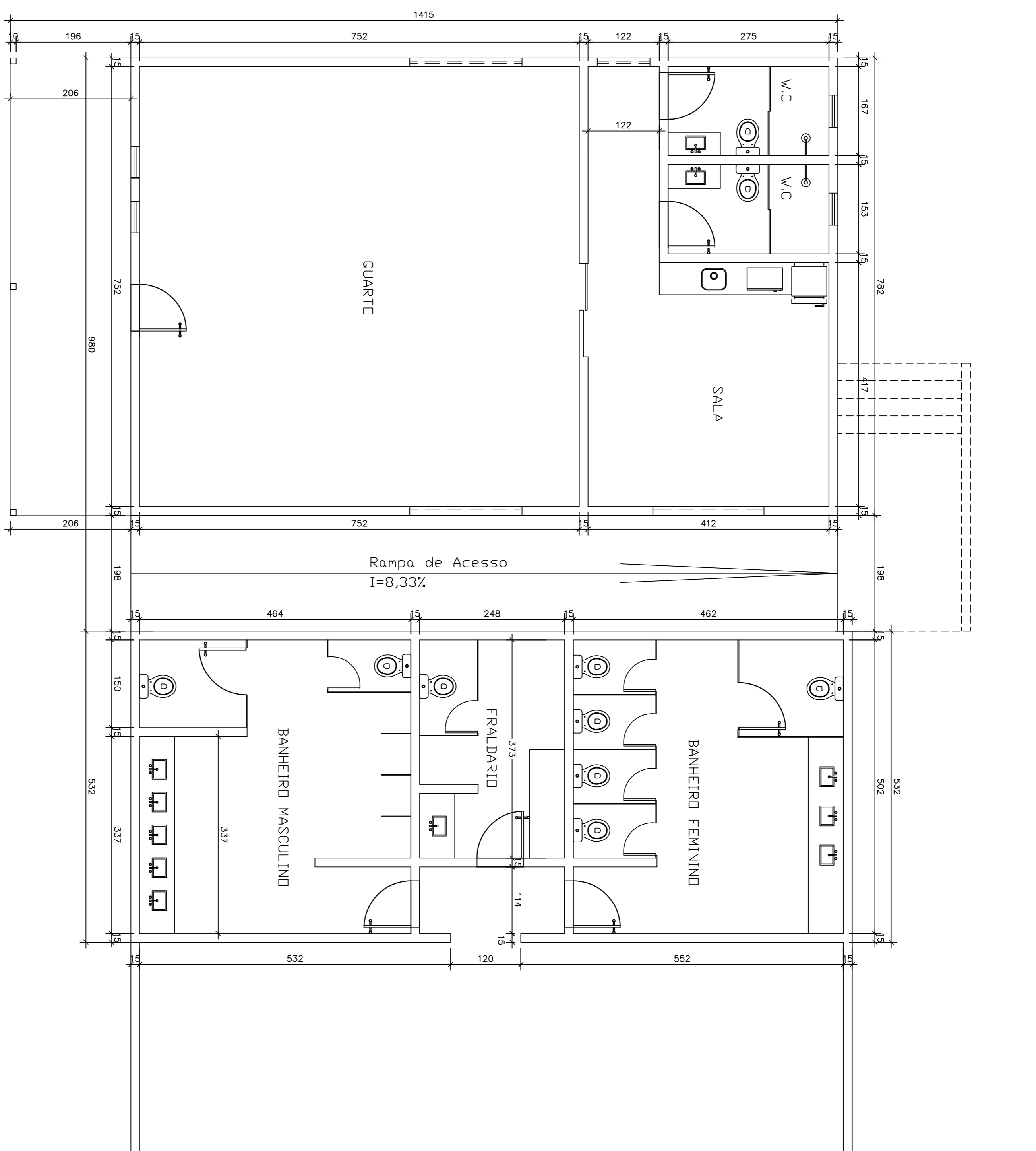
PLANTA ÁREA DE LAZER escala 1/50
